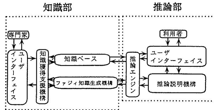
Fig. 1 法律ファジィエキスパートシステムの構成
