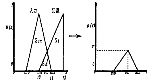
Fig. 3 入力と知識のマッチング
