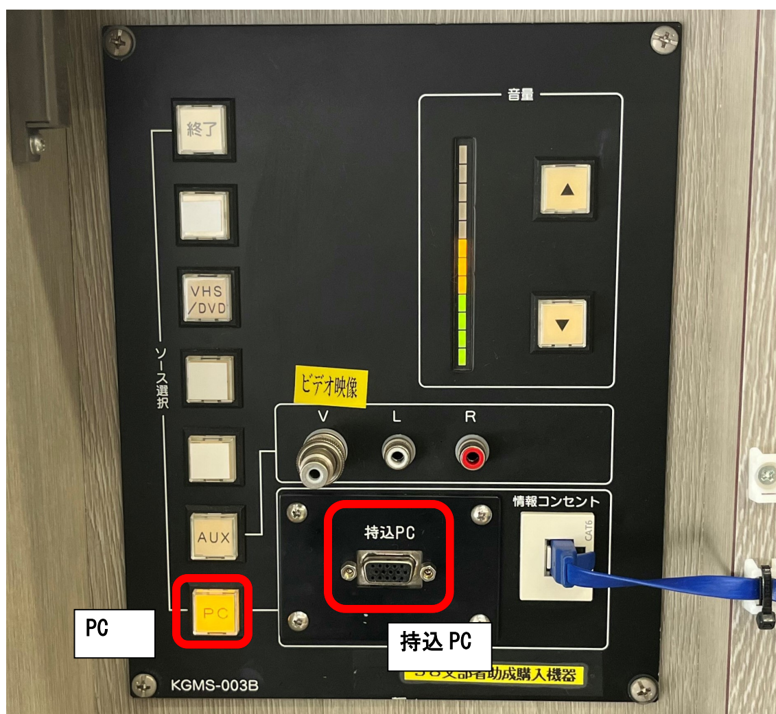
図1. 操作盤
